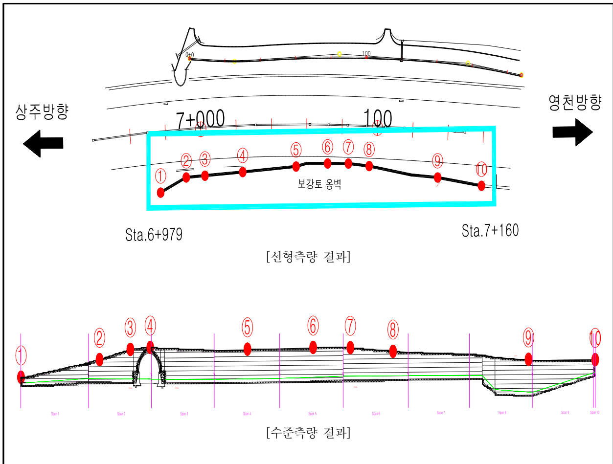
【그림 9.3.5】 선형 및 수준측량 결과
